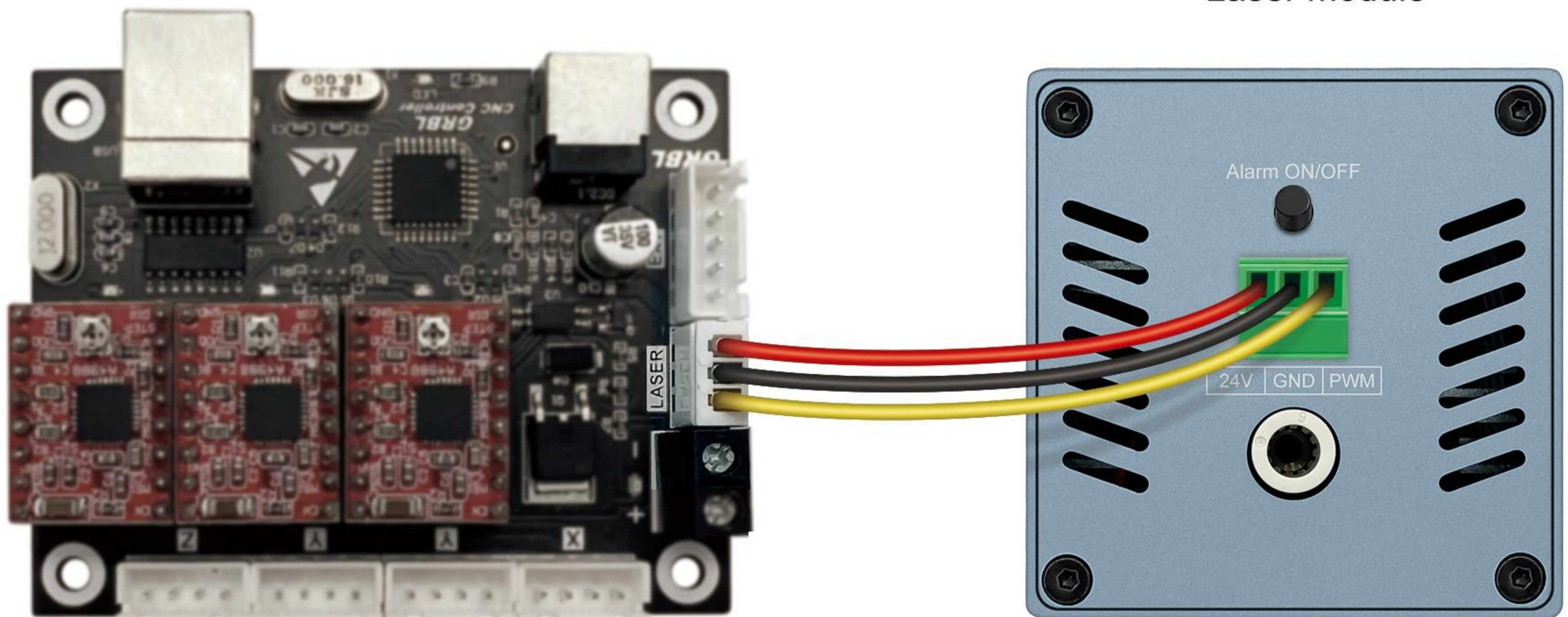
Laser module
